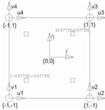
Rys. 3. Element czworoboczny 4-węzłowy i funkcje kształtu
