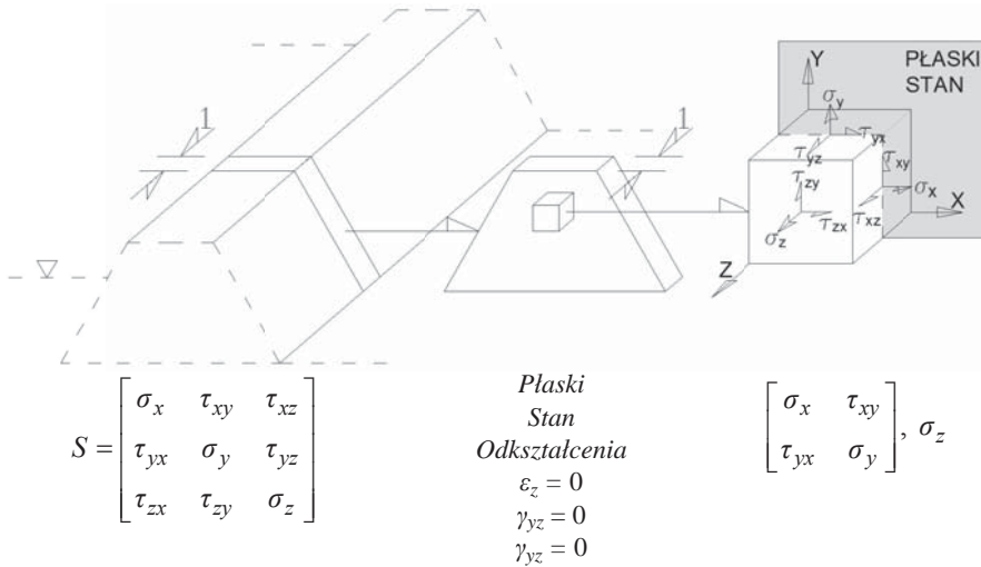
Rys. 5. Warunki płaskiego stanu odkształcenia dla przykładu wału przeciwpowodziowego podanego parciu wody i redukcja tensora naprężenia do płaskiego stanu
