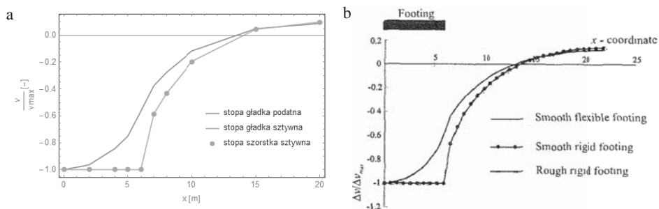
Rys. 7. Przemieszczenia powierzchni terenu: a – obliczenia własne dla elementu 4-węzłowego, b – obliczenia Potts i Zdravkovic [1999] dla elementów 8-węzłowych
