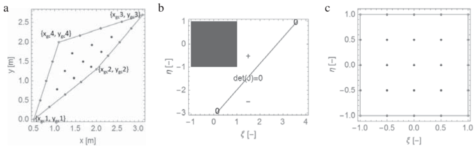
Rys. 4. Procedura zmiany współzrędnych 4-węzłowego, czworobocznego elementu skończonego: a – element we współzrędnych globalnych, b – linia zerowego Jakobianu, c – element we współzrędnych bezwymiarowych lokalnych
