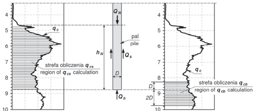
Rys. 2. Schemat obliczania ekwiwalentnych wartości oporów stożka q_{cs} i q_{cb} .
