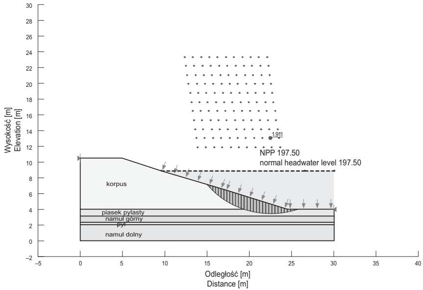
Rys. 3. Stateczność zapory w Nieliszu przy NPP (197,50 m n.p.m.) Fig. 3. The stability of the Nielisz dam at reservoir level (197.50 m)
