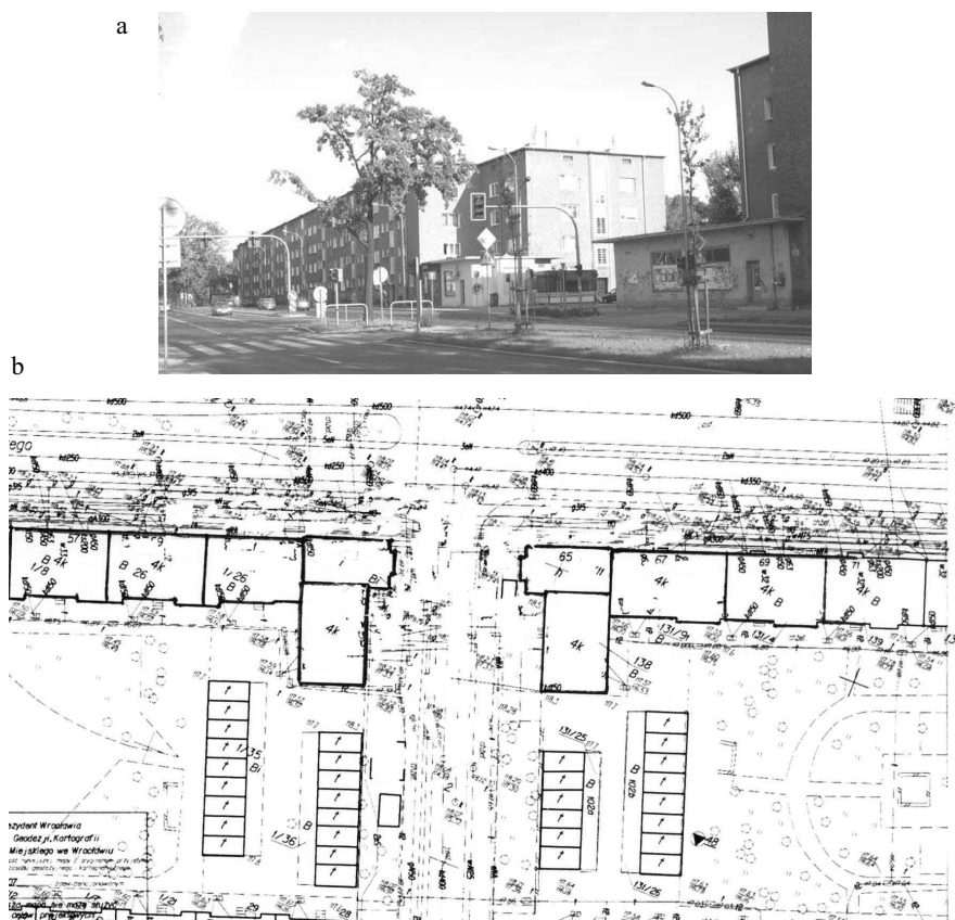
Rys. 11. Modernistyczna zabudowa we Wrocławiu, narożne domy przy ul. Bolesława Krzywoustego (około 1930 r.): a – widok, b – plan
