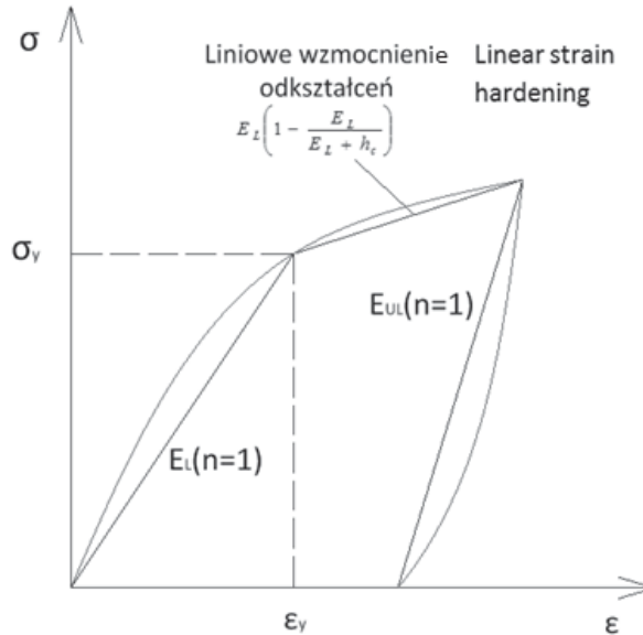
Rys. 1. Pierwszy cykl obciążania wraz z uproszczonym modelem P-D
